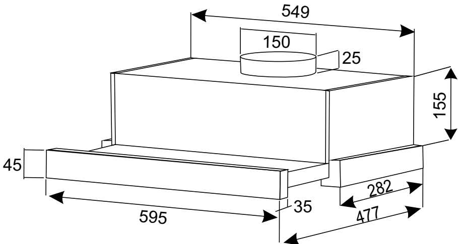
Рис. 8 Схема монтажа вытяжки
